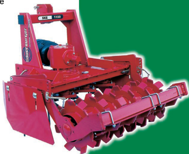
SKE 1150 s rozměňovacím "packer" válcem
